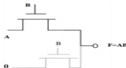
Fig.4. PTL Circuit
