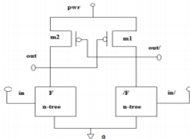
Fig.2. ECRL
