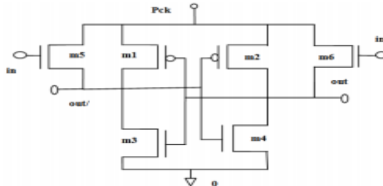
Fig.3. PFAL
