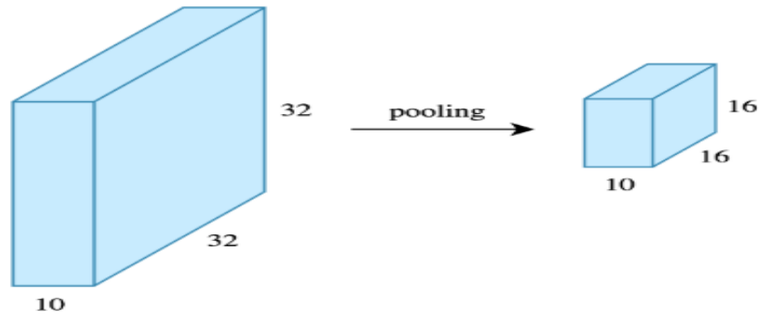
Fig. 3 Pooling layer
