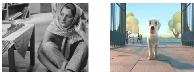
Fig. 3: Stego image.
