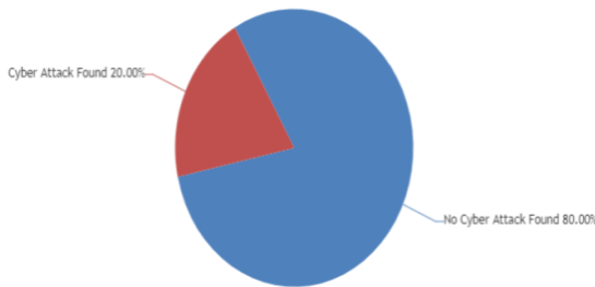
Fig. 13: Venn Diagram
