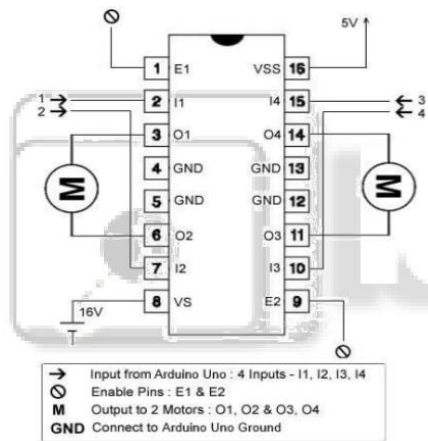
Fig. 7: L293D IC
