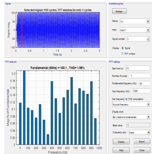
Fig.9. THD values.
