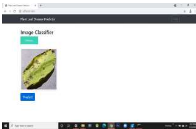
Fig.4.2. INPUT image.
