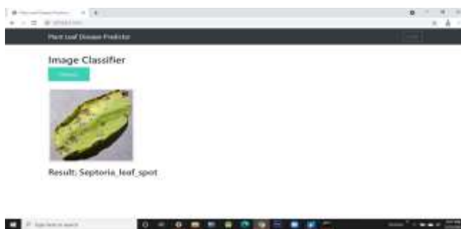
Fig.4.3. OUTPUT image.
